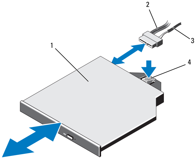
그림 3-16. 광학 드라이브 분리 및 설치
