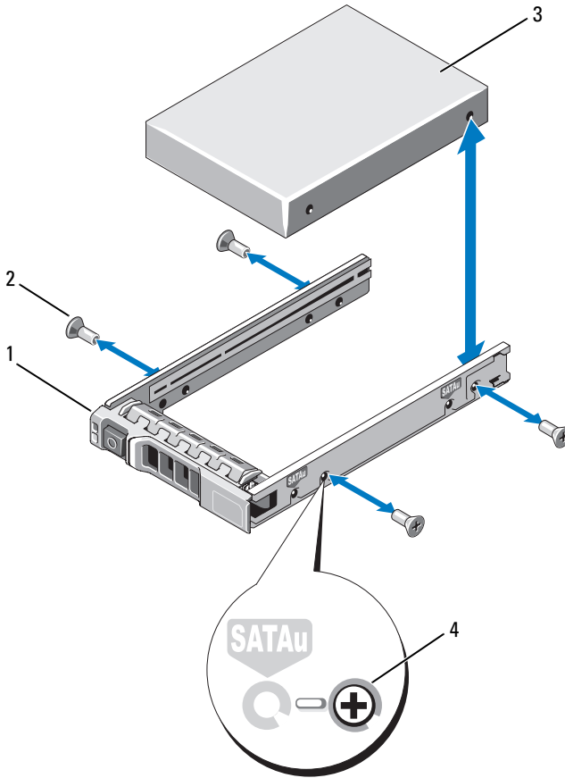
그림 3-7. 드라이브 캐리어에 하드 드라이브 설치
