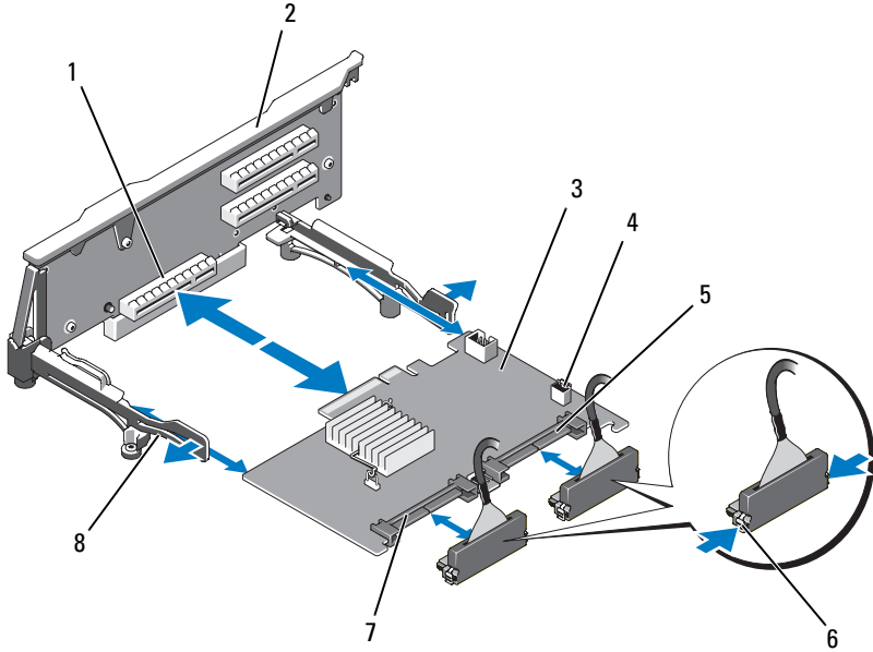
그림 3-18. 저장 컨트롤러 카드 설치
