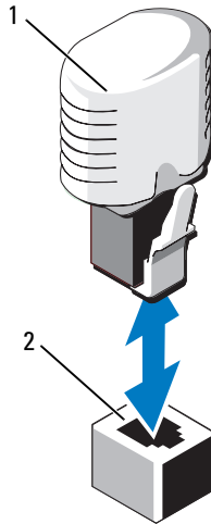
1 NIC 하드웨어 키 2 ICSI_KEY 커넥터
