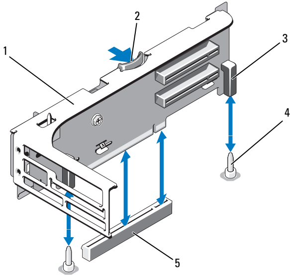
그림 3-24. 확장 카드 라이저 2 분리 및 장착
