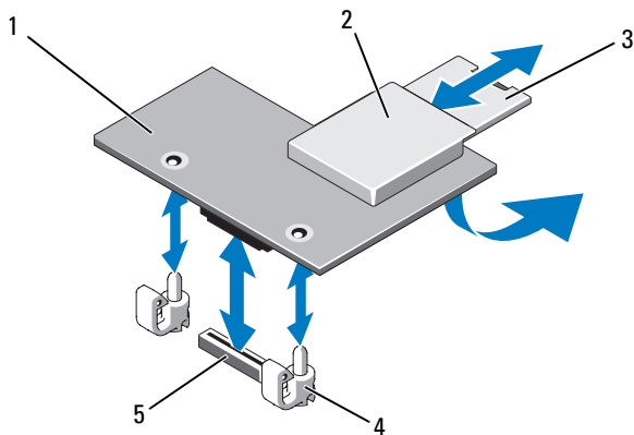
그림 3-11. iDRAC6 Enterprise 카드 분리 및 설치
