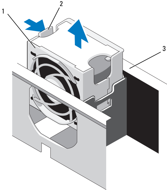
그림 3-14. 냉각 팬 분리 및 설치
