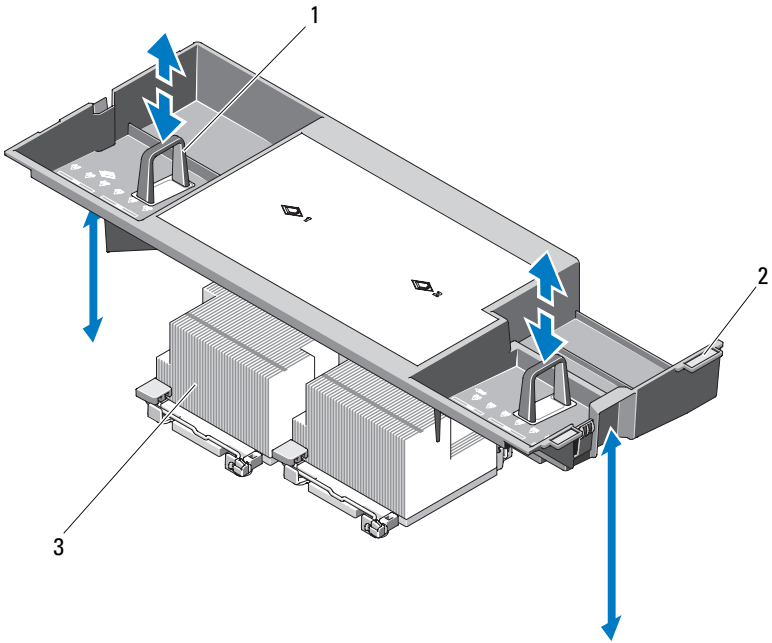
그림 3-13. 냉각 덮개 분리 및 설치
