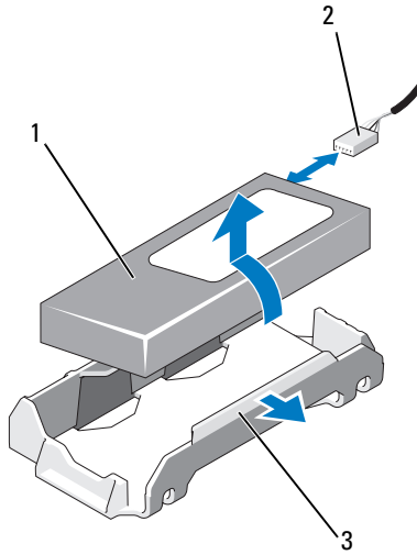
그림 3-20. RAID 배터리 분리 및 설치
