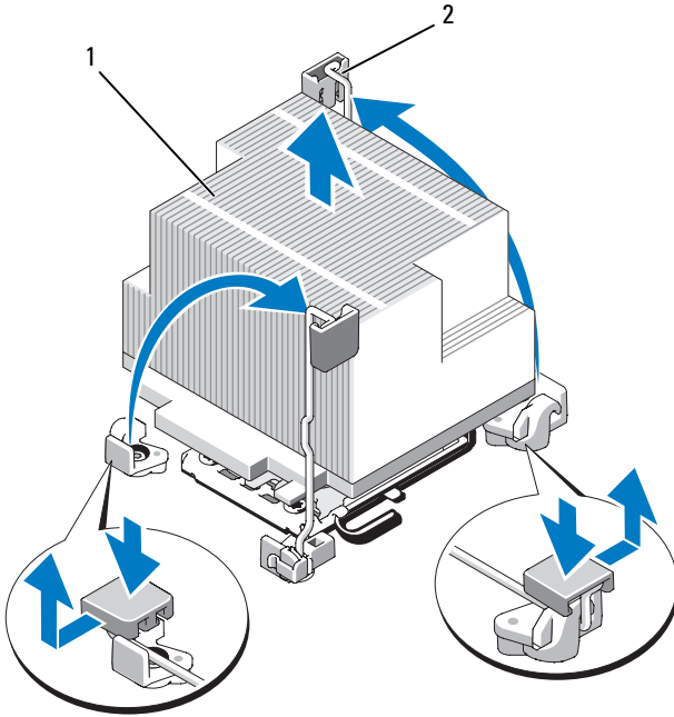
1 방열판 2 분리 레버 (2 개)
