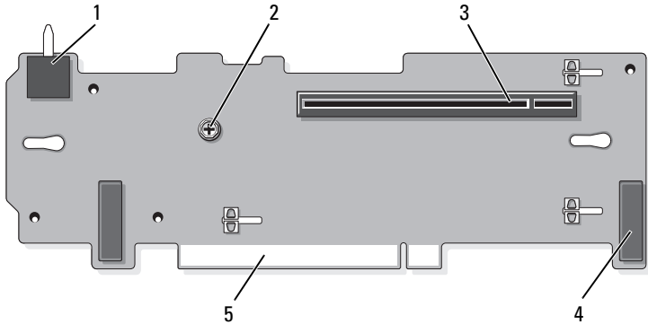
그림 6-6. PCIe x16 확장 카드 라이저 2 구성요소 (선택 사양)
