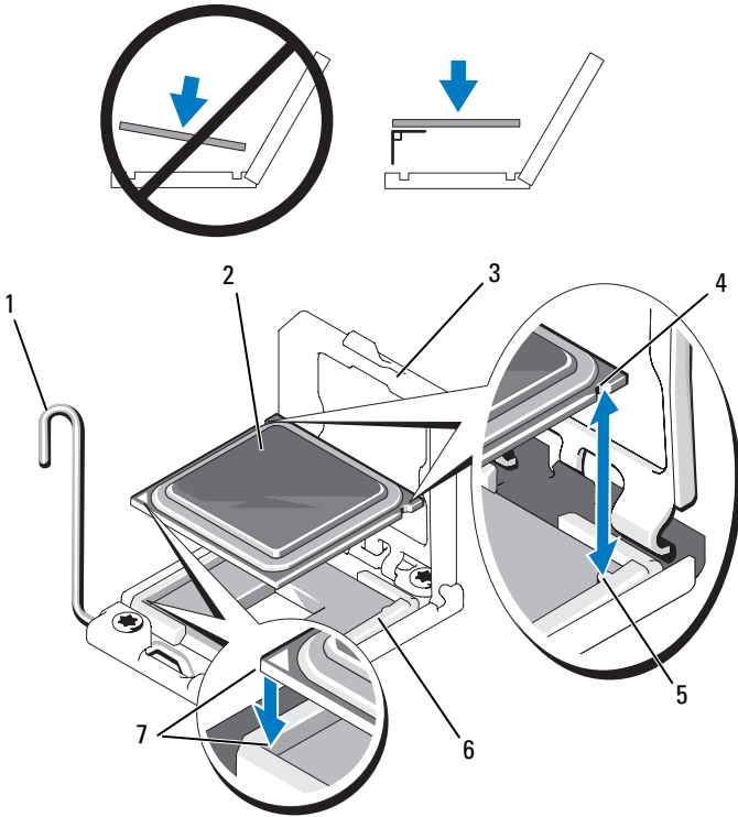
그림 3-29. 프로세서 설치 및 분리
