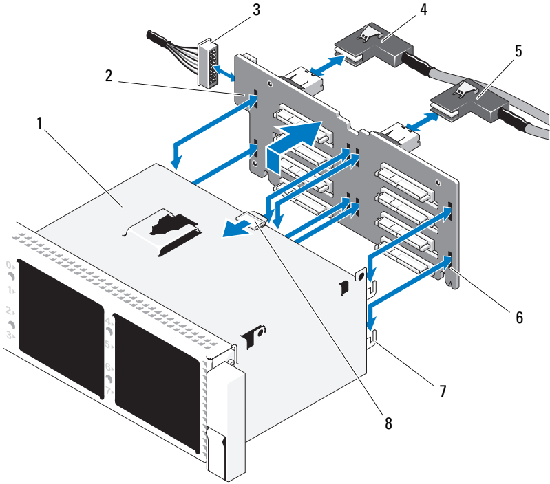
그림 3-33. SAS 후면판 분리 및 설치
