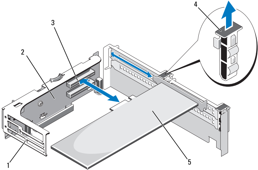
그림 3-22. 확장 카드 분리 또는 설치
