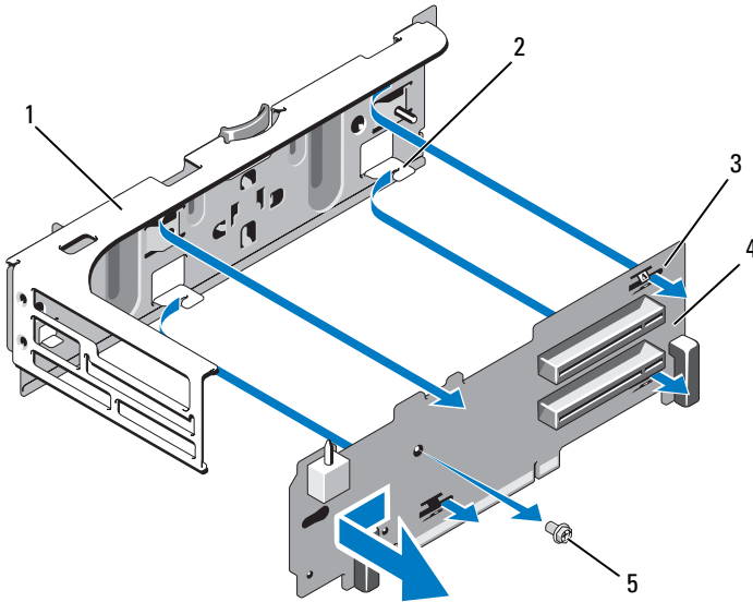
그림 3-25. 라이저 2 보드 분리 및 장착
