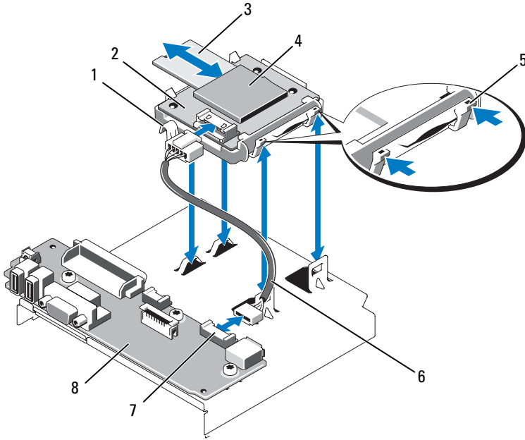
그림 3-9. 내부 SD 모듈 분리 또는 설치
