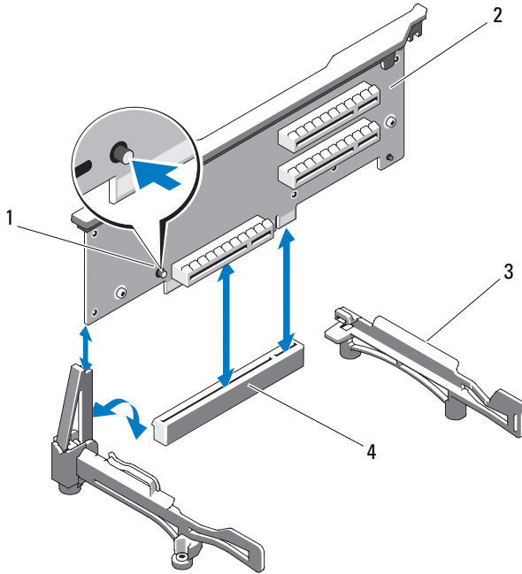
그림 3-23. 확장 카드 라이저 1 분리 및 장착
