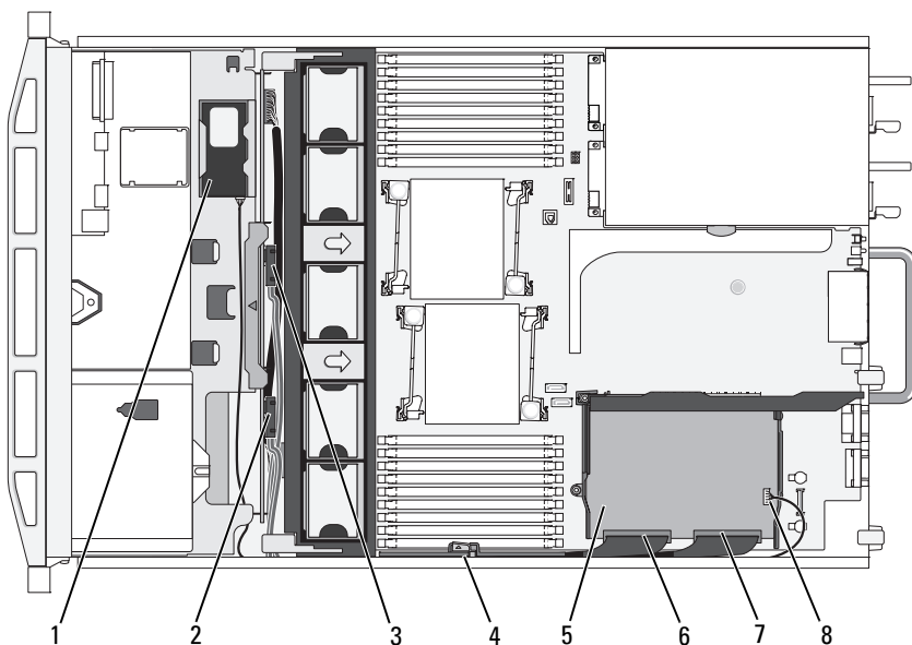
그림 3-19. 스토리지 컨트롤러 카드 케이블 연결
