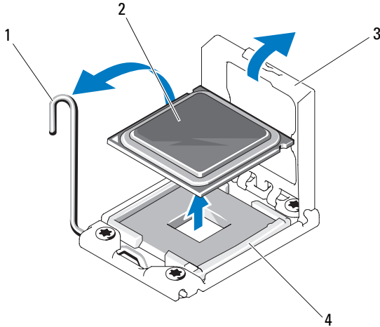
그림 3-28. 프로세서 분리
