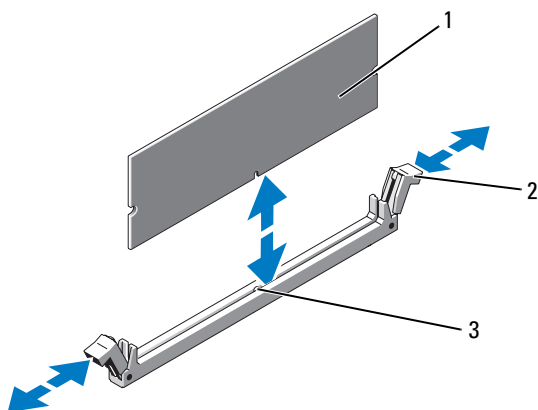
그림 3-26. 메모리 모듈 설치 및 분리
