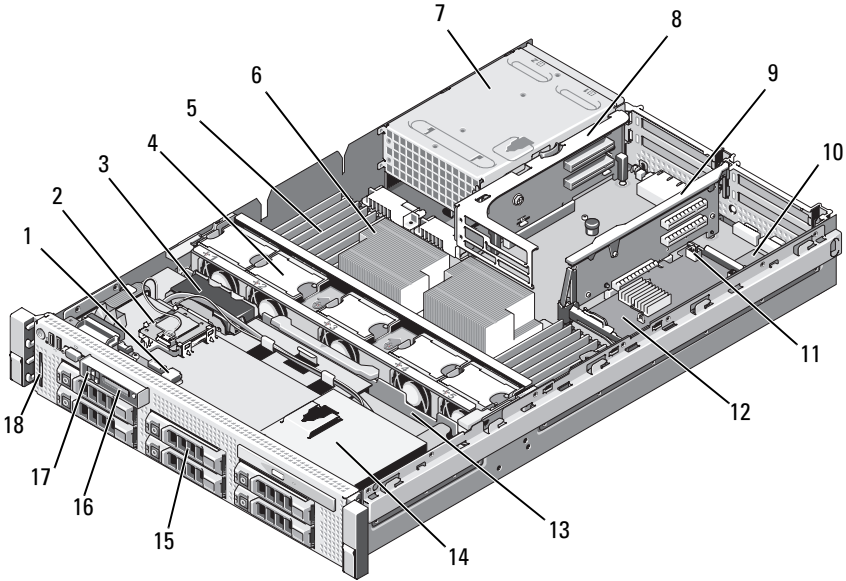
그림 3-1. 시스템 내부
