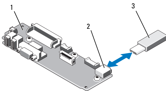
그림 3-10. USB 메모리 키 분리 또는 설치
