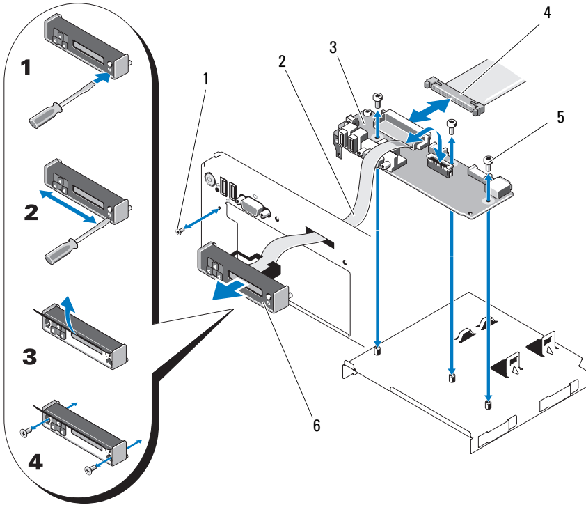
그림 3-32. 제어판 분리 및 설치
