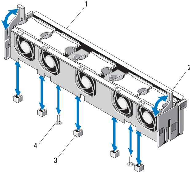
그림 3-15. 프로세서 팬 브래킷 분리 및 설치
