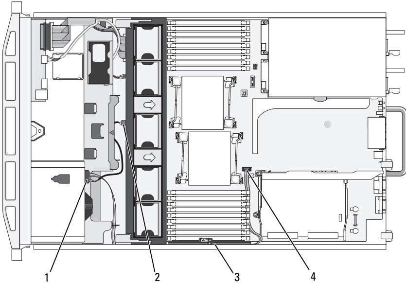
그림 3-17. 광학 드라이브 케이블 경로 지정
