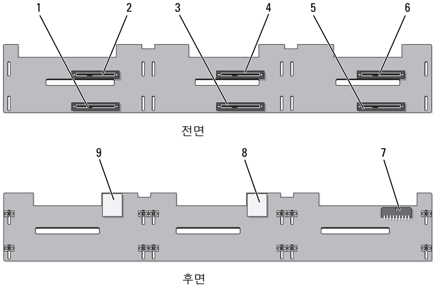
그림 6-3. SAS 후면판 보드 (6 슬롯 )
