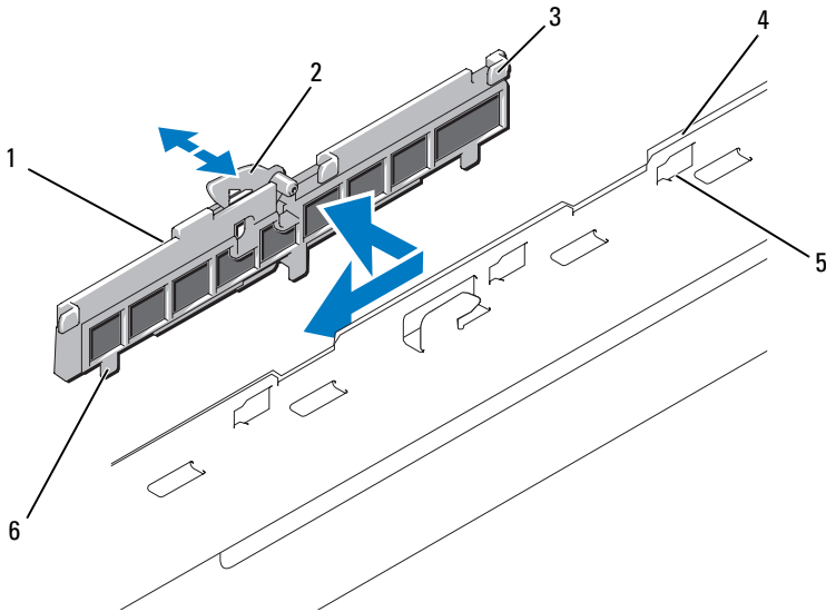
그림 3-21. 케이블 고정 브래킷 분리 및 설치
