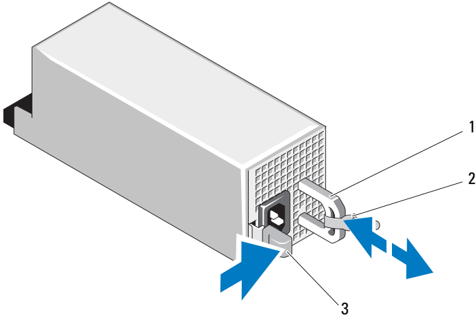
그림 3-8. 전원 공급 장치 분리 및 설치
