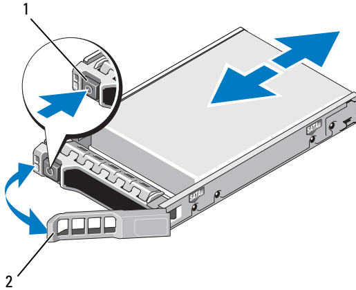
1 분리 단추 2 하드 드라이브 캐리어 핸들
